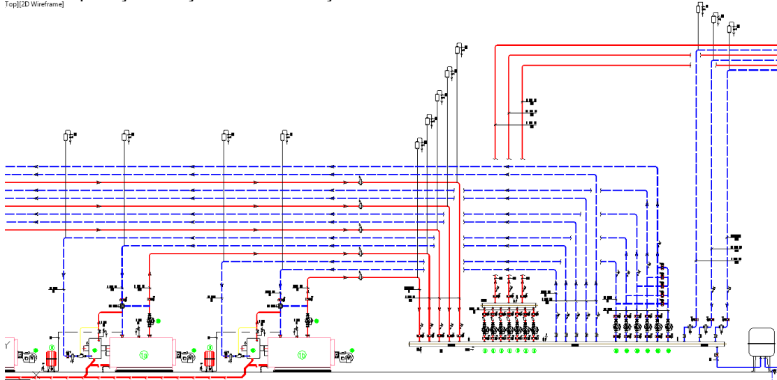
Şekil 2. Kazan dairesinde hidrolik denge kontrollü tek kolektörlü dağıtım sistemi
