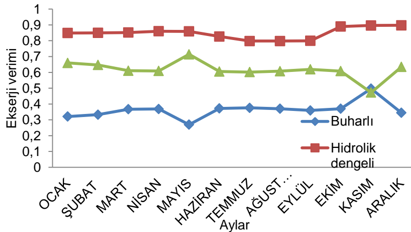
Şekil 4. Yerleşkenin karşılaştırmalı ekserji verimi ve dağılımı
