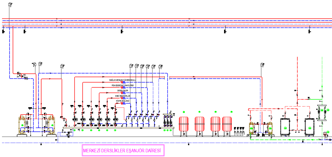
Şekil 3. Eşanjör dairesinde hidrolik denge kontrollü tek kolektörlü dağıtım sistemi
