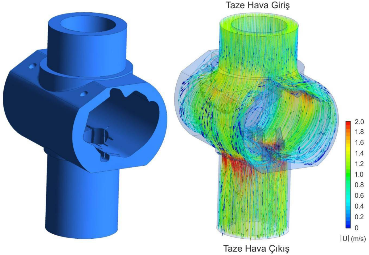
Şekil 5.2.7. Dış kasa simülasyon modeli (sağ resim) ve üç boyutlu akış çizgileri (sol resim)
