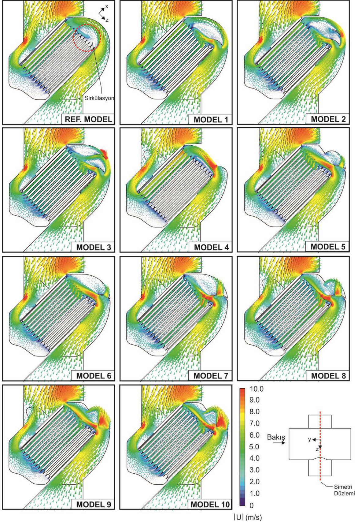
Şekil 5.2.3. Simetri düzlemi üzerindeki üç boyutlu hız vektörleri
