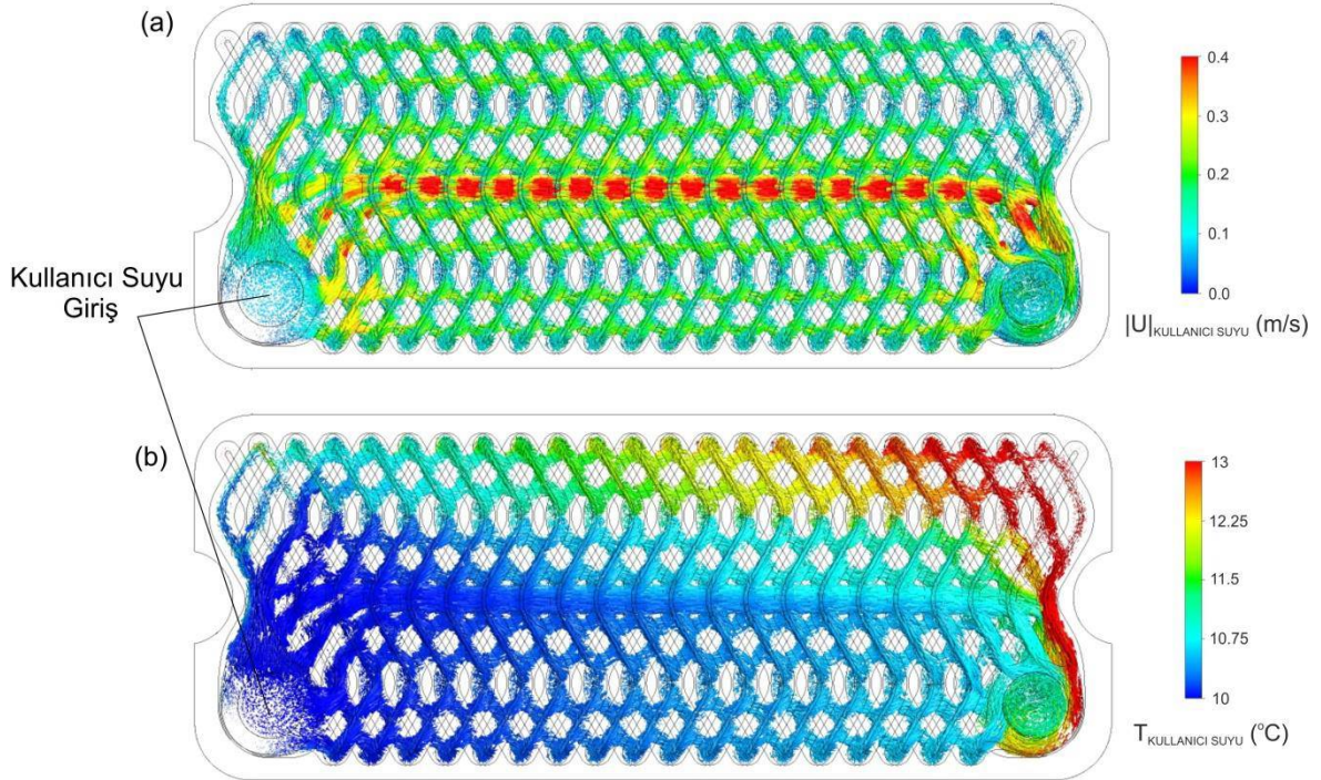
Şekil 5.1.2. Kullanıcı suyu 3 boyutlu hız vektörlerinin hız büyüklüğü (a), ve sıcaklık (b) ile gösterilmesi.
