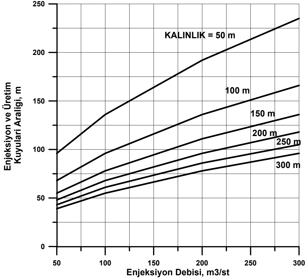
Şekil 8. Suyun 8 ay boyunca sabit debide basılması durumunda ısı kirlenmenin oluşmaması için gerekli güvenilir aralığın formasyon kalınlığı ve enjeksiyon debisiyle ilişkisi.
