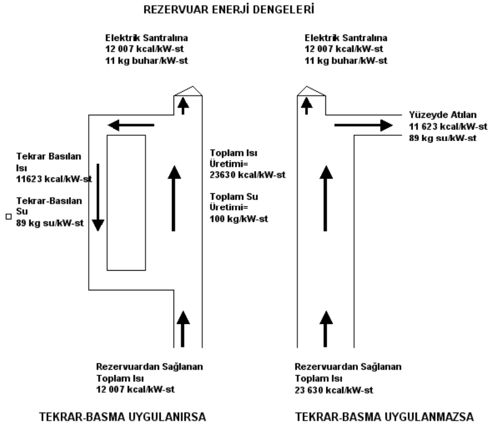
Şekil 13. 10 MW elektrik santrali için tekrar-basma uygulanırsa (solda) ve uygulanmayipta atık su yüzeyde harcanırsa (sağda) rezervuarda enerji dengeleri. (Satman v.ö., 1997)
