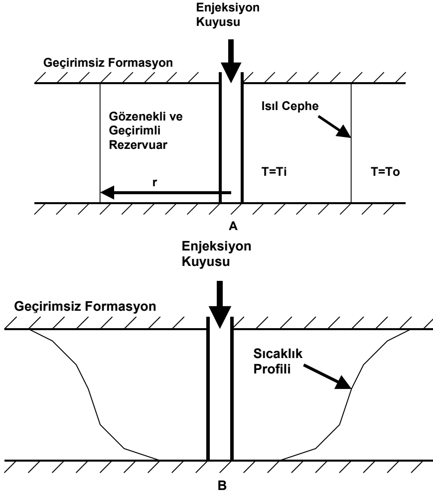
Şekil 2. Başlangıç sıcaklığı T_0 olan gözenekli ortama T_i sıcaklığında çevrel akışta su basılmasında oluşan sıcaklık dağılımı: ( a) Alt ve üstteki geçirimsiz formasyonlara ısı geçişi olmaması durumu b) Alt ve üstteki geçirimsiz formasyonlara ısı geçişi olması durumu.)
