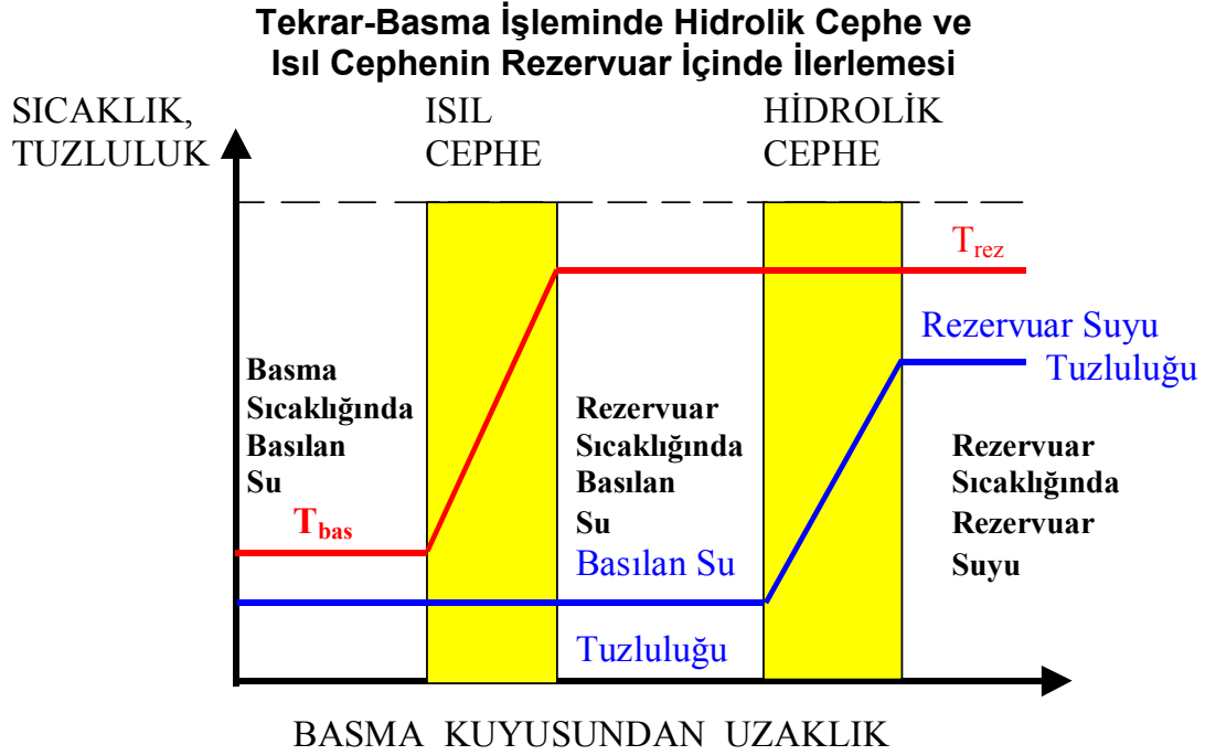
Şekil 1. Tekrar-basma işleminde hidrolik cephe ve ısıl cephenin rezervuar içinde ilerlemesi.
