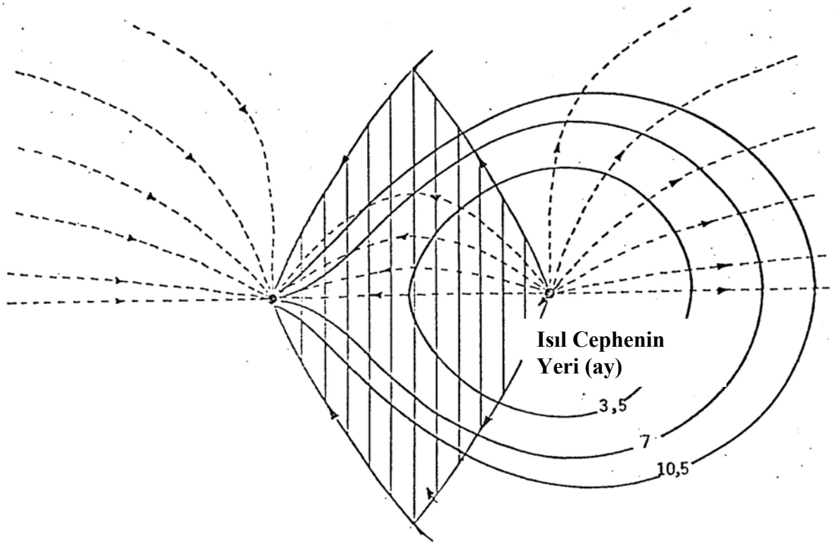
Şekil 3. Kuyu çifti modeli için kesik çizgiler akış çizgilerini gösterirken, kesiksiz çizgiler 3.5, 7 ve 10.5 ay enjeksiyon sonunda ısı cepheyi göstermektedir.
