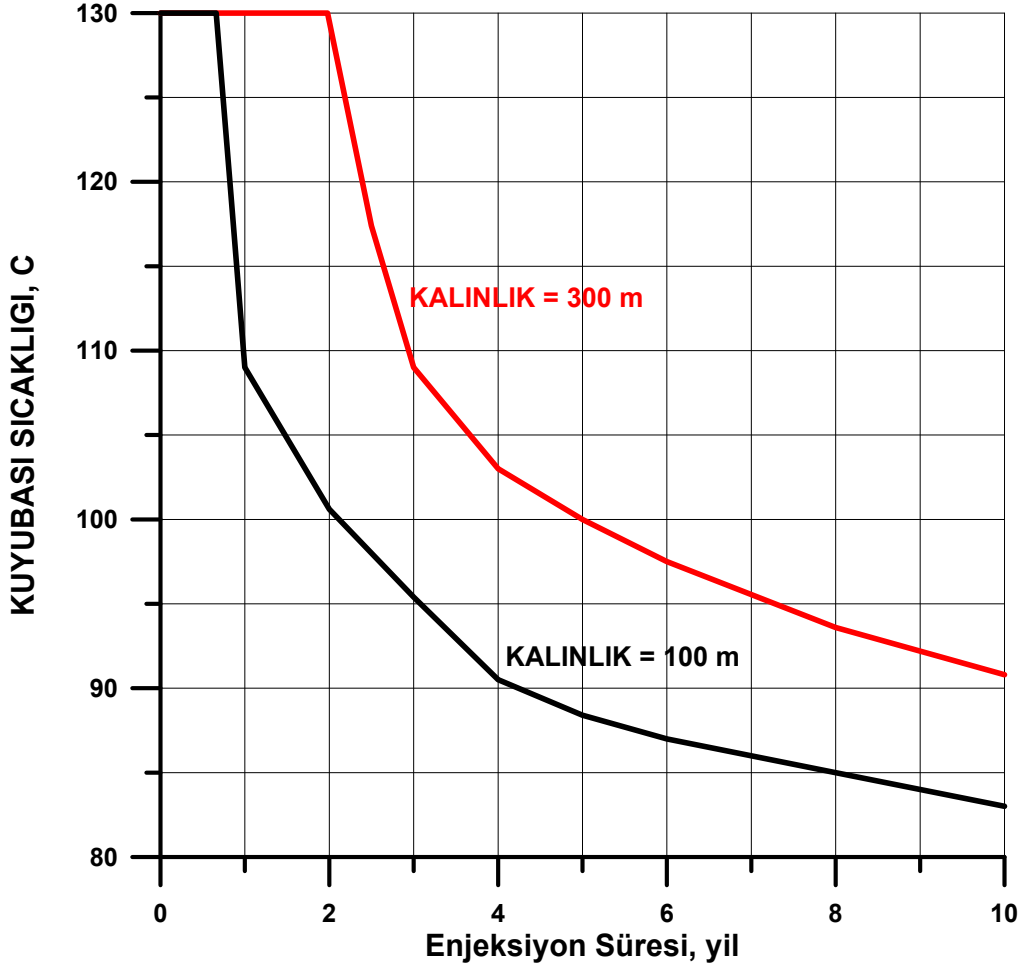
Şekil 9. Enjeksiyon ve Üretim kuyuları arasında 100 m aralık bulunması ve suyun 108 m 3 /st debide basılması durumunda kuyubaşı üretim sıcaklığının enjeksiyon süresi ile değişimi.
