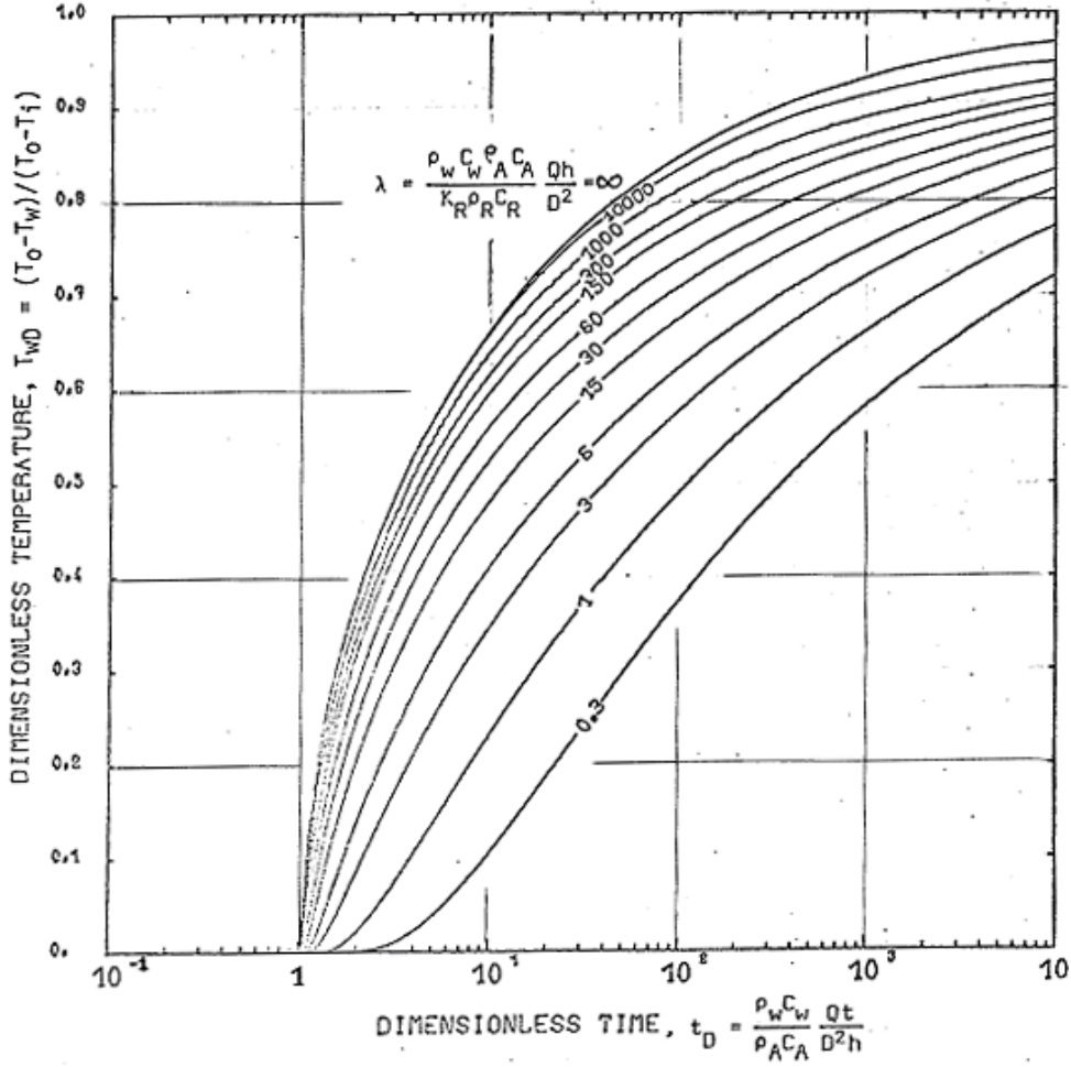
Şekil 4. Kuyuçifti modelinde rezervuar içinde sıcaklık dağılımını bulmakta kullanılan Gringarten-Sauty (1975) grafiği.
