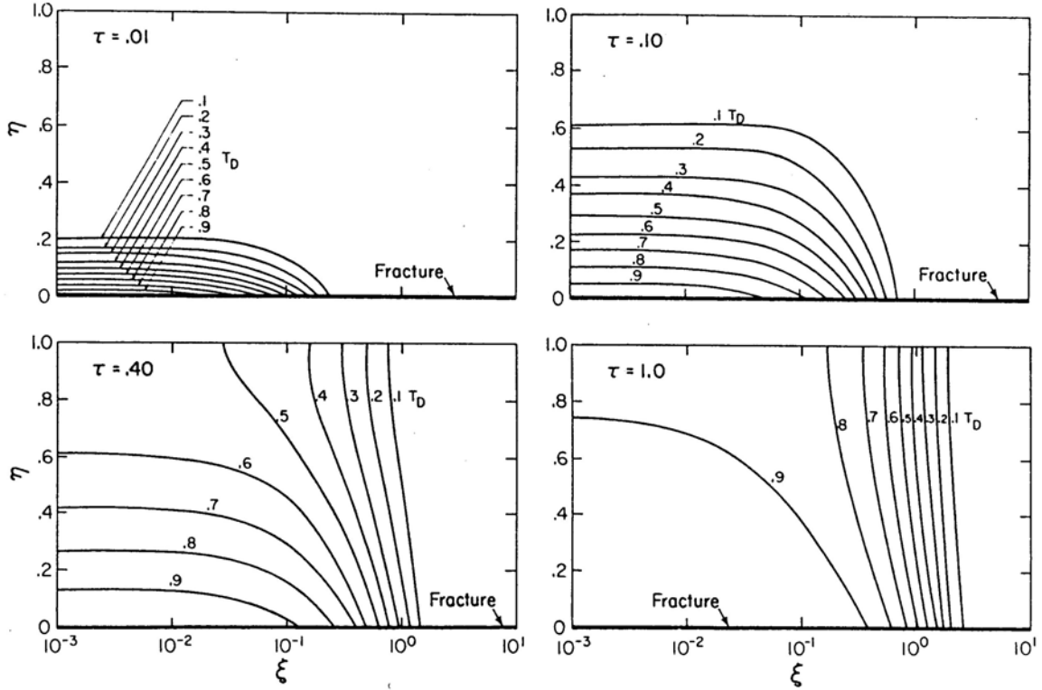
Şekil 6. Çatlaklı bir rezervuarda farklı enjeksiyon zamanlarında sistem içinde sıcaklık dağılımları. (Bodvarsson ve Tsang, 1981)
