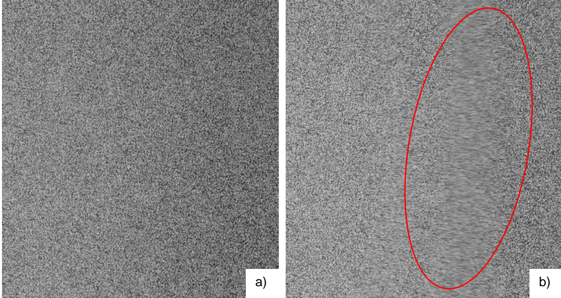
Şekil 2. a) Deneyin başlamasından önce çekilen referans fotoğrafı b) Deney sırasında çekilen akış görüntüleme fotoğrafı
