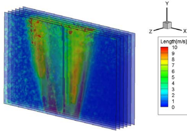
Şekil 7. Sıcak jet akış üzerinden alınan düzlemsel PGHÖ görüntüleri
