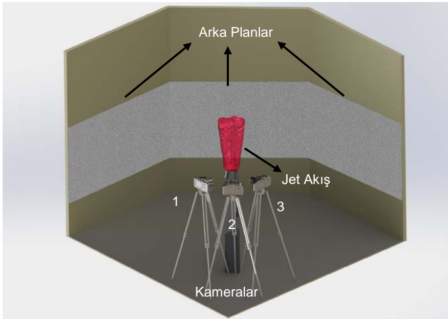
Şekil 4. Üç boyutlu arka plan konumlandırılmış yoğunluk farkı yönteminin şematik gösterimi
