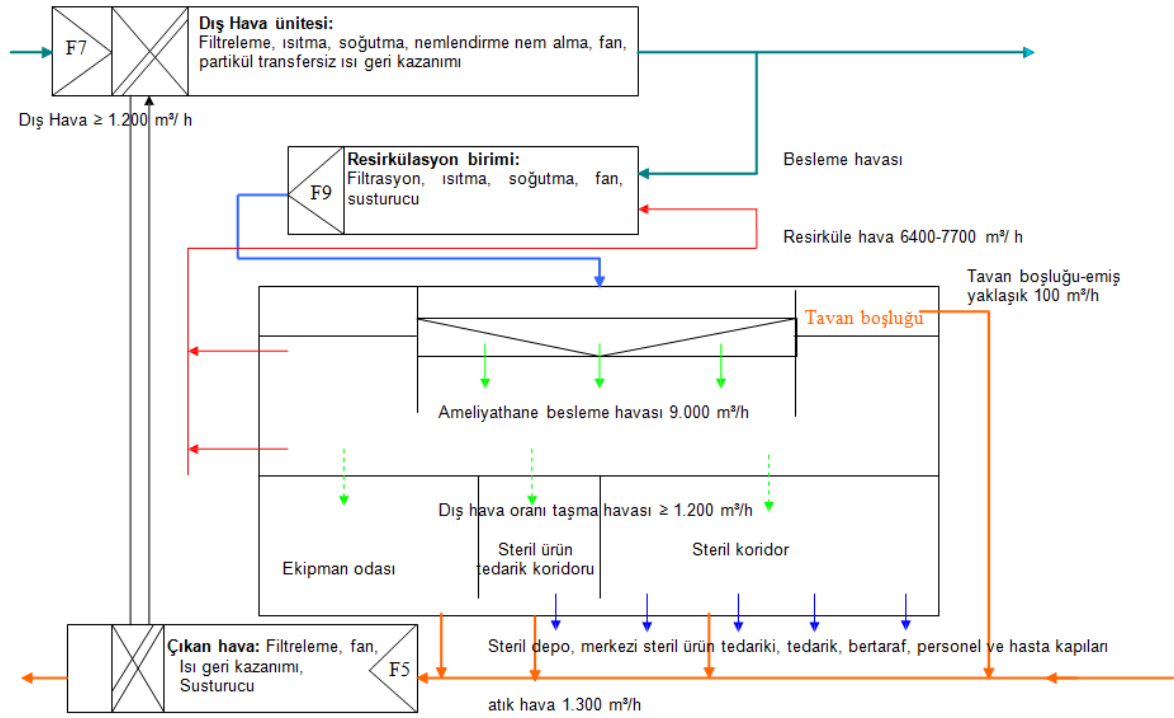
Şekil 2. Düşük türbülanslı doğrusal akışlı besleme havası tavanı için sistem prensip şeması (oda sınıfı Ia) [3]
