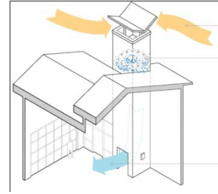
Çağdaş Sistemde Buharlaştırma ile Doğal Havalandırma The Global Ecology Center in Standford, California, USA[18].
