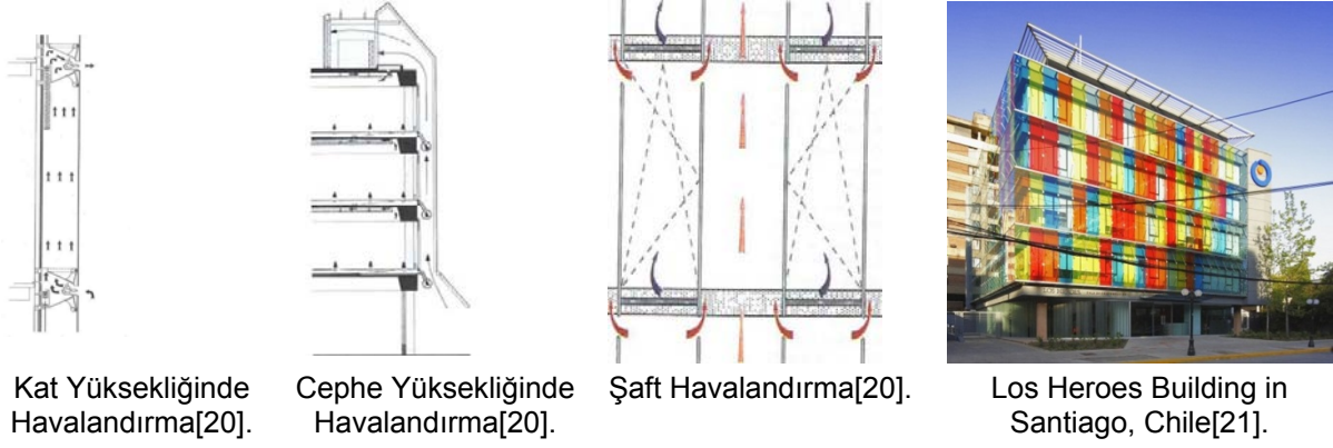
Şekil 3. Çift Cam Cephe
