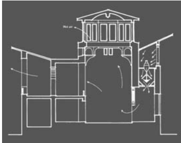
Geleneksel Yöntemde Buharlaştırma ile Doğal Havalandırma [18].
