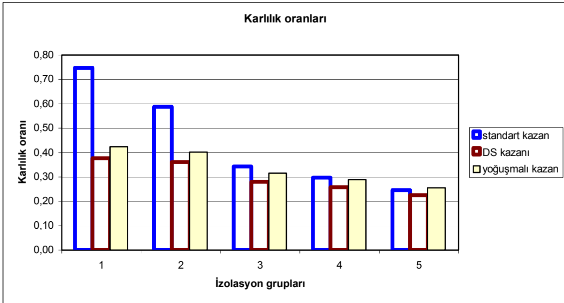
Şekil 10. Karlılık oranlarının mevcut bina için ahşap çerçeveli tek camlı pencere ve termostatik vanalı durumda farklı izolasyon kalınlık alternatifleri ve farklı kazan hallerindeki değişimi
