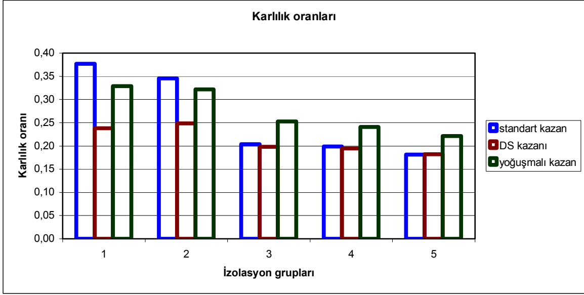
Şekil 9. Karlılık oranlarının mevcut bina için ahşap çerçeveli tek camlı pencere ve termostatik vanasız durumda farklı izolasyon kalınlık alternatifleri ve farklı kazan hallerindeki değişimi
