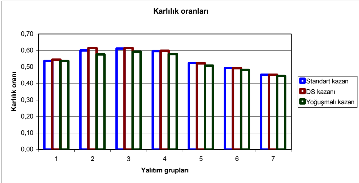
Şekil 6. Contalı plastik çerçeveli çift camlı pencere ve termostatik vanalı durumda farklı izolasyon kalınlık grupları ve farklı kazan hallerindeki karlılık oranları
