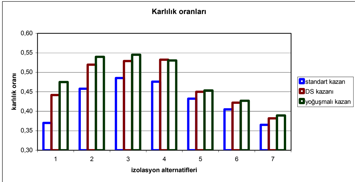
Şekil 4. Karlılık oranlarının ahşap çerçevli tek camlı pencere ve termostatik vanasız durumda farklı izolasyon kalınlık alternatifleri ve farklı kazan hallerindeki değişimi
