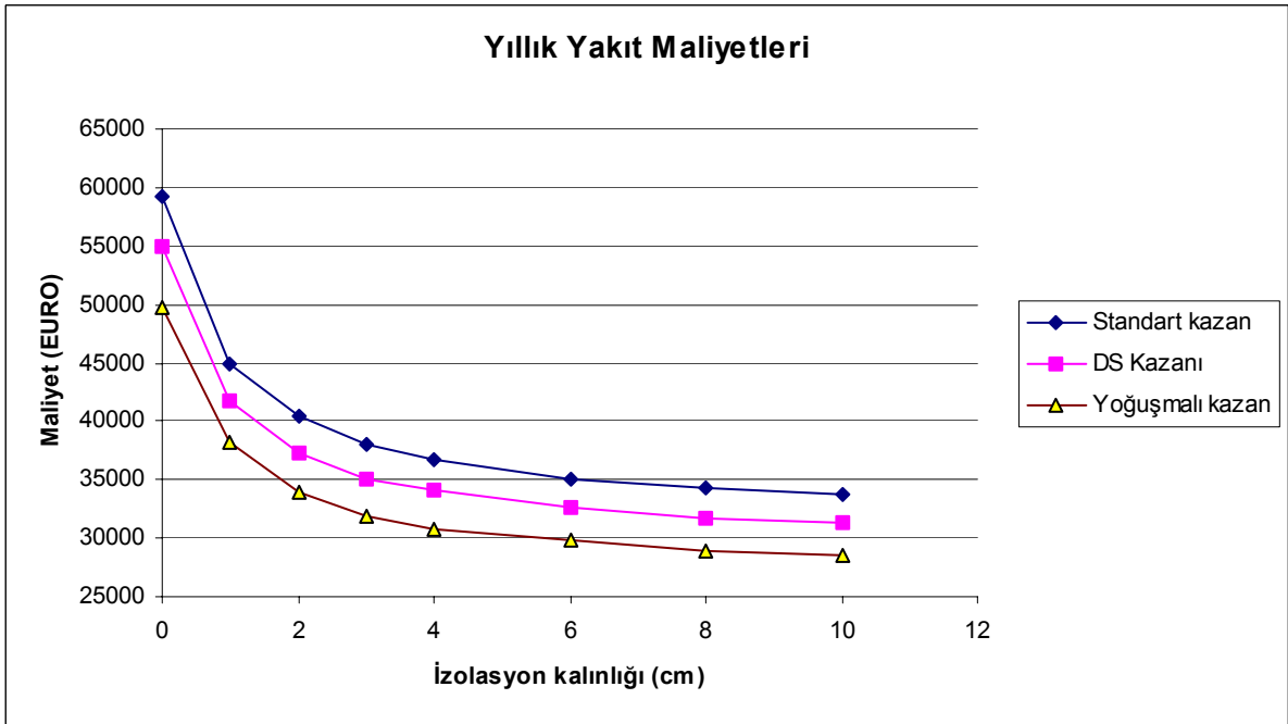
Şekil 3. Yıllık yakıt maliyetlerinin ahşap çerçeveli tek camlı pencere ve termostatik vanasız farklı izolasyon kalınlıkları ve farklı kazan hallerindeki değişimi
