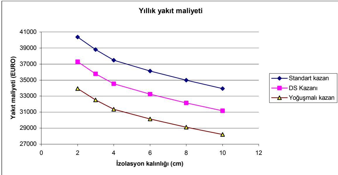
Şekil 8. Yıllık yakıt maliyetlerinin mevcut binada ahşap çerçeveli tek camlı pencere ve termostatik vanasız durumda farklı izolasyon kalınlıkları ve farklı kazan hallerindeki değişimi
