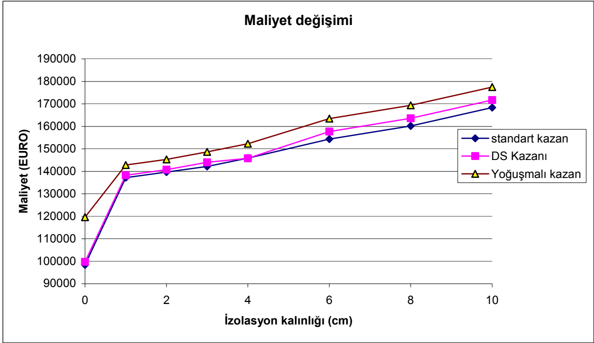
Şekil 2. Yeni bina için yatırım maliyetlerinin ahşap çerçeveli tek camlı pencere ve termostatik vanasız halde farklı izolasyon kalınlıkları ve farklı kazan tipleri için değişimi
