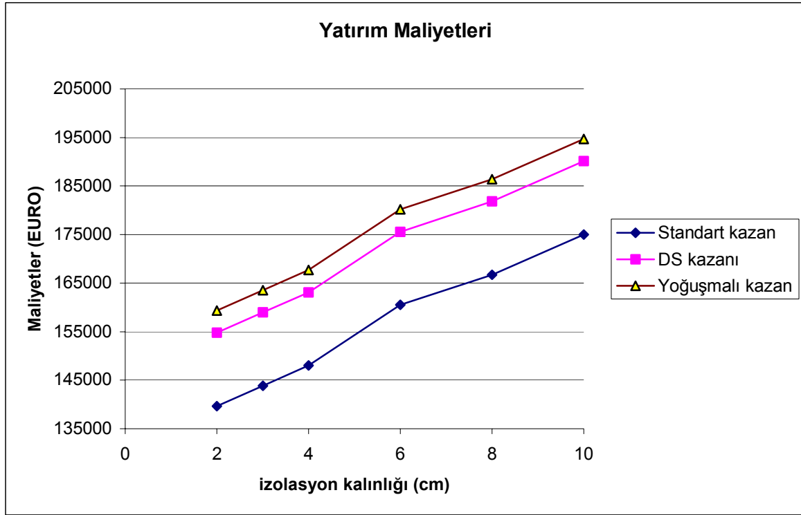
Şekil 7. Mevcut binada yatırım maliyetlerinin, ahşap çerçeveli tek camlı pencere ve termostatik vanasız hal için, farklı izolasyon kalınlıkları ve farklı kazan hallerindeki değişimi
