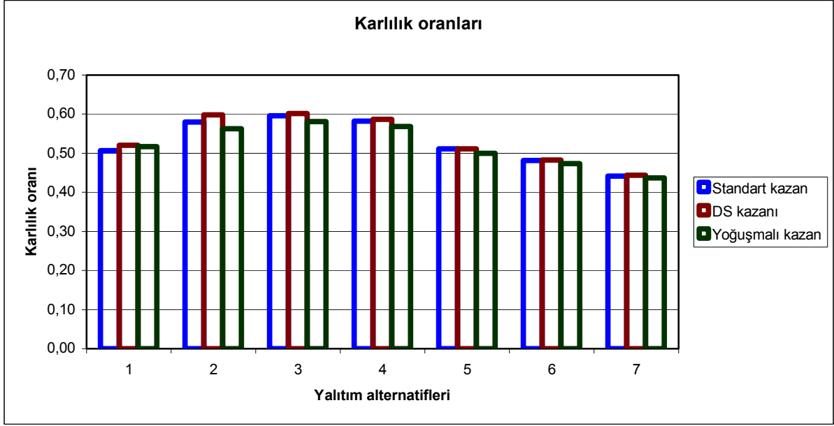
Şekil 5. Karlılık oranlarının contalı plastik çerçeveli çift camlı pencere ve termostatik vanasız durumda farklı izolasyon kalınlık alternatifleri ve farklı kazan hallerindeki değişimi
