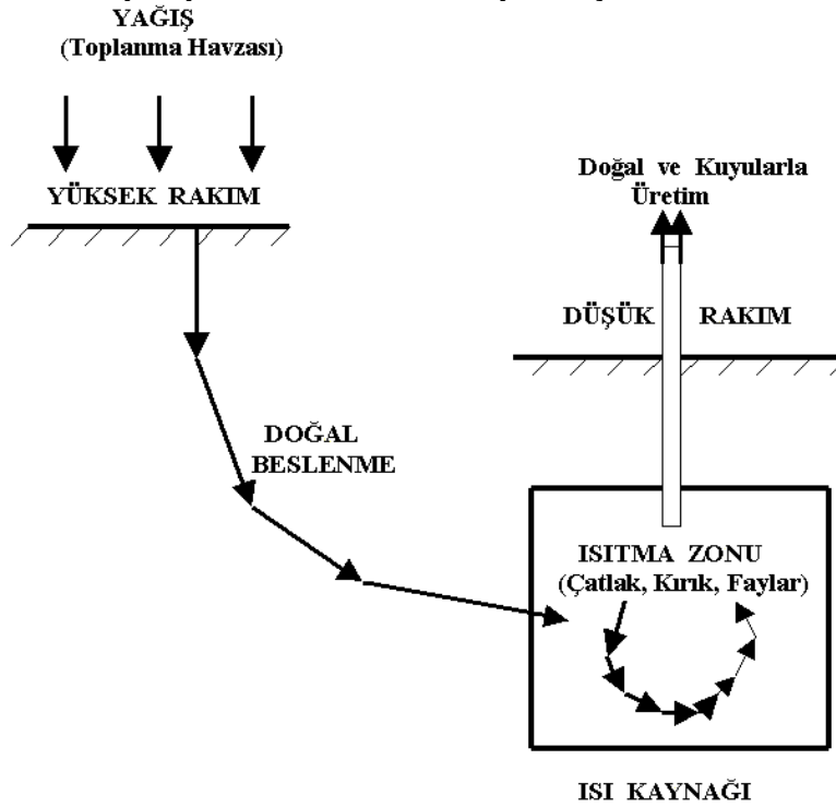
Şekil 1. Düşük sıcaklıklı sistemler için ısı kaynağı mekanizması modeli
