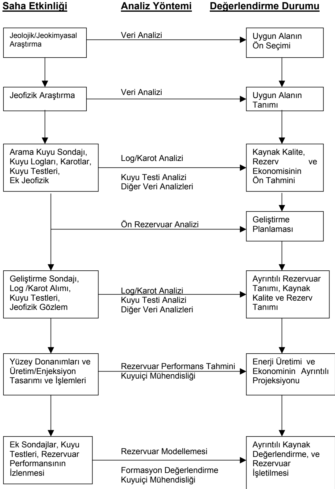
Şekil 4. Jeotermal rezervuar (kaynak) deđerlendirme akış şeması.
