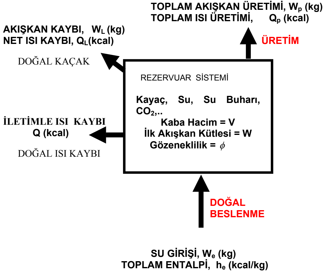
Şekil 5. Boyutsuz rezervuar modeli.
