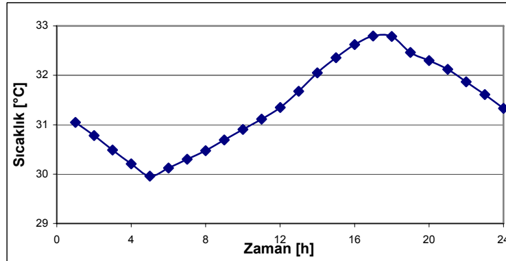
Şekil 6. Tipik Bina için İç Ortam Sıcaklık Değerleri
