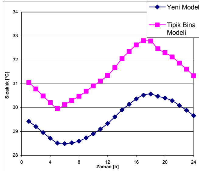
Şekil 8. Pencere özelliklerinin ortam sıcaklığı üzerindeki etkisi
