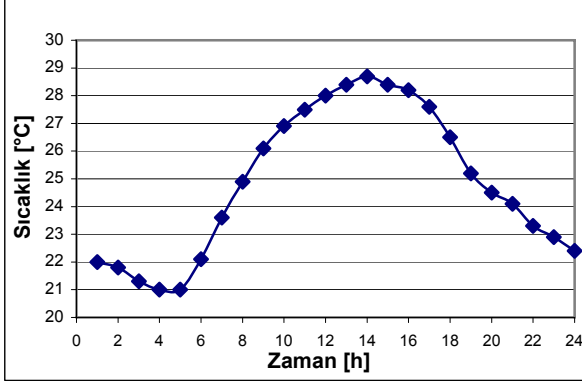
Şekil 4. 21 Temmuz günü, İstanbul iklimi için dış ortam sıcaklıkları
