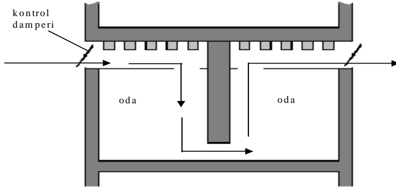
Şekil 9. Doğal havalandırma için tasarlanan bina yapısı
