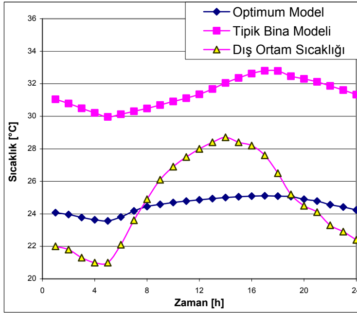
Şekil 11. Doğal soğutma için tasarlanan optimum modelin sıcaklık değişimleri
