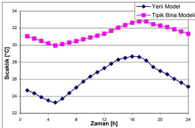
Şekil 10. Enfiltrasyonun ortam sıcaklığı üzerindeki etkisi
