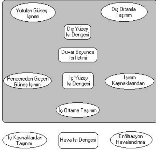
Şekil 1. Bir bina yapı elemanı için ısı dengesi
