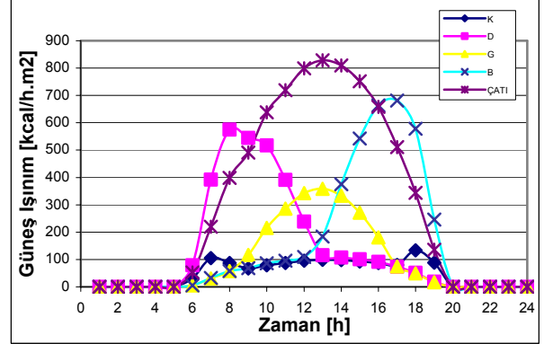
Şekil 5. 21 Temmuz günü, İstanbul iklimi için güneş ışınımı değerleri.
