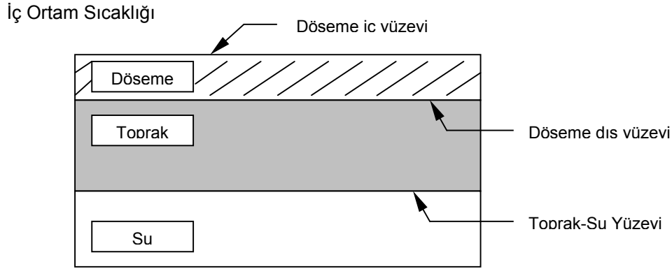
Şekil 3. Oluşturulan döşeme modeli
