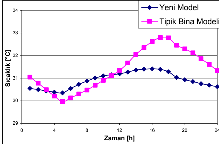
Şekil 7. Bina yapı özelliklerinin ortam sıcaklığı üzerindeki etkisi
