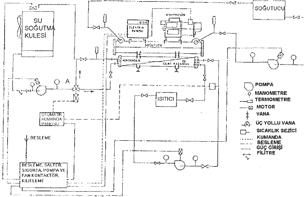
SU SOĞUTMALI KONDENSERLİ ISI GERİ KAZANIMLI CİHAZ VE EKİPMANLARI PRENSİP ŞEMASI
