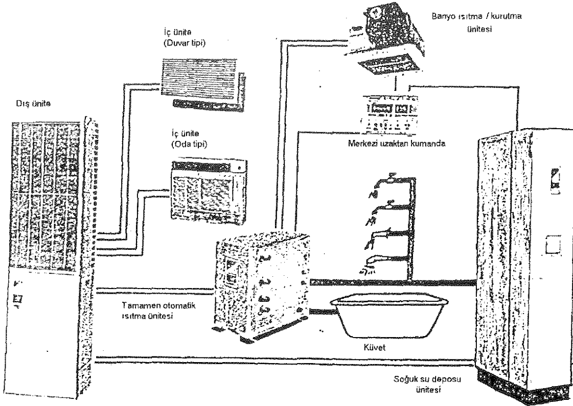
Daikin "Trilo System" çok fonksiyonlu evsel kullanım sistemi
