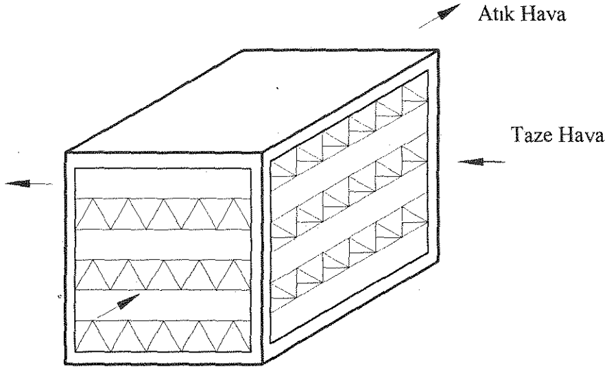
Şekil 8. Levhalı ısı eşanjörü
