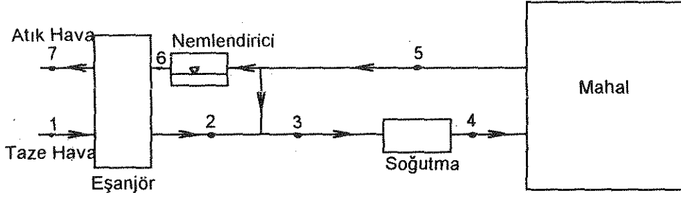
Şekil 17. Isı geri kazanımında nemlendiricili yaz kliması
