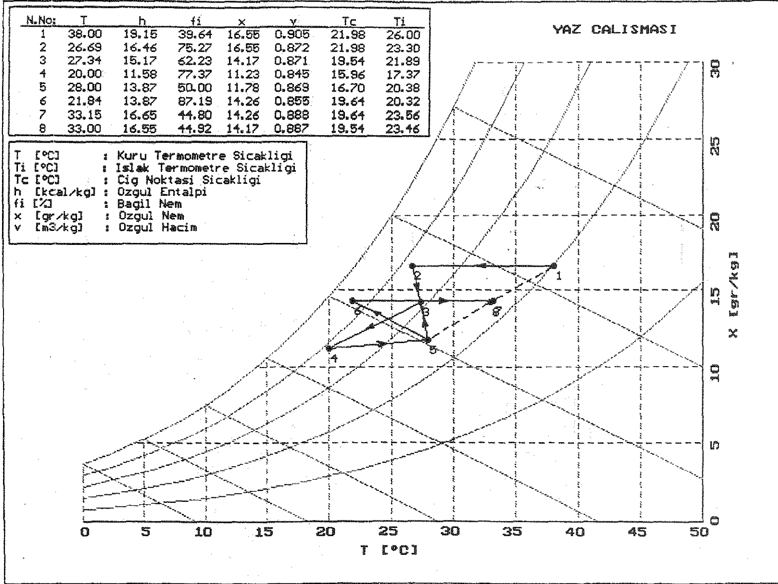
Şekil 18. Işı geri kazanımlı nemlendiricili yaz ikliminin psikrometrik diyagramda gösterilişi
