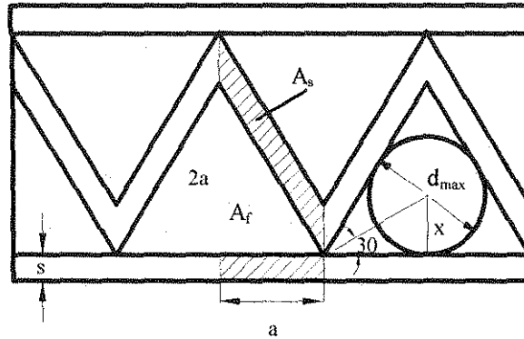
Şekil 6. Kanal geometrisi
