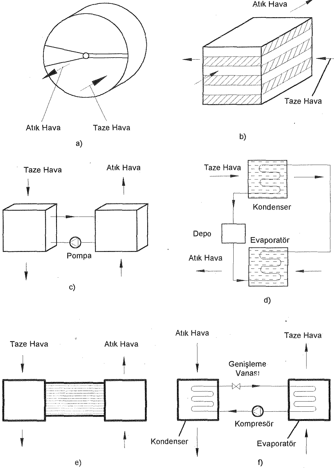
Şekil 2. Çeşitli enerji geri kazanım sistemleri
