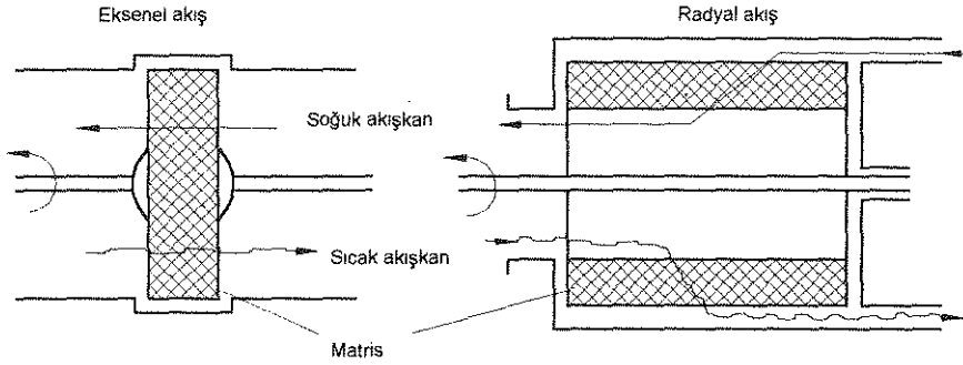
Şekil 4. Döner rejeneratör tipleri a) Disk tipi, b) Tambur tipi
