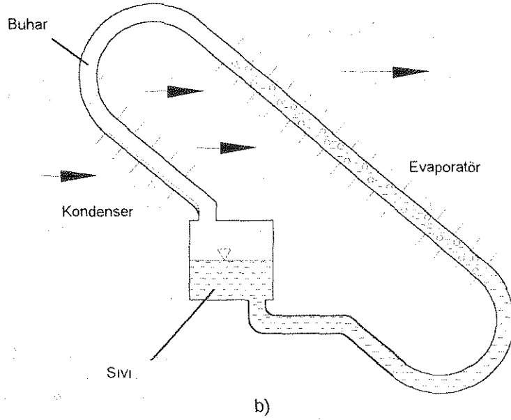
Şekil 10. Çift fazlı çift eşanjörlü sistemler
