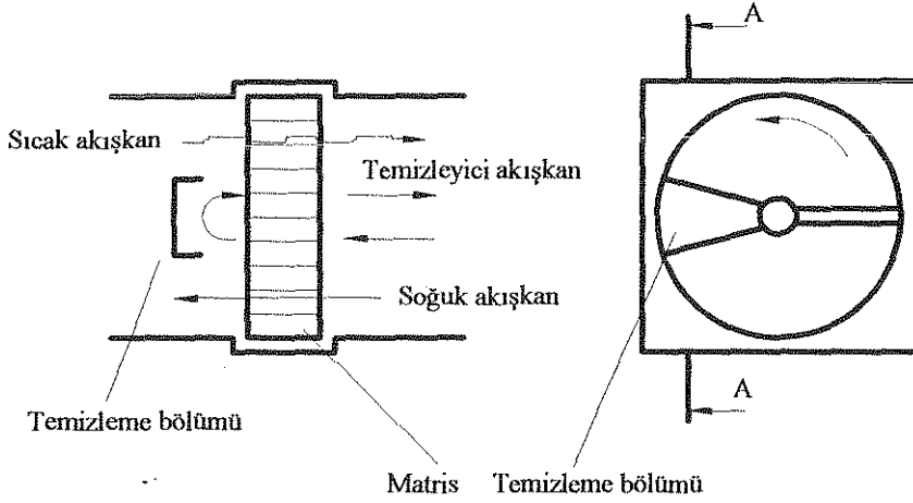
Şekil 3. Döner rejeneratör
