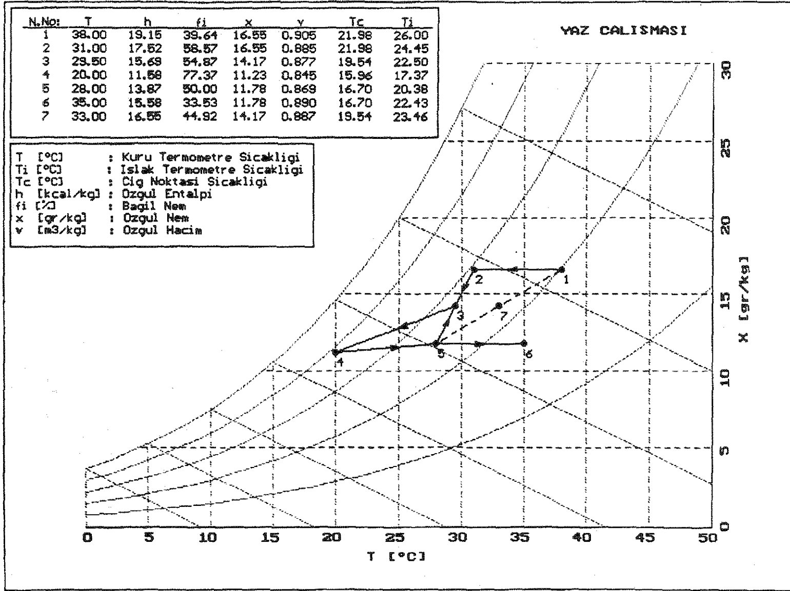
Şekil 16. Isı geri kazanımlı nemlendiricisiz yaz ikliminin psikrometrik diyagramda gösterilişi
