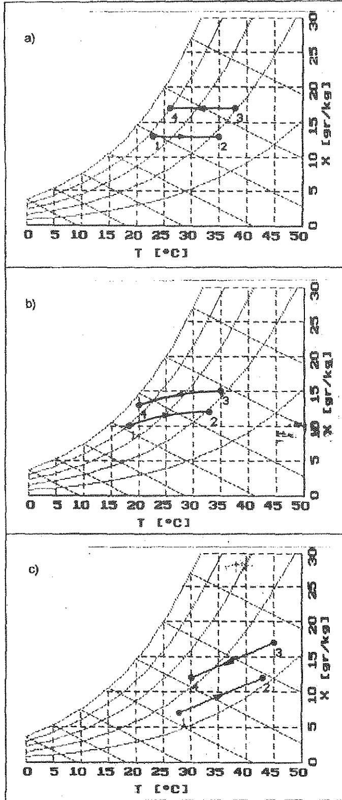
Şekil 1. Isı eşanjörlerindeki havanın psikrometrik diyagramda gösterimi
