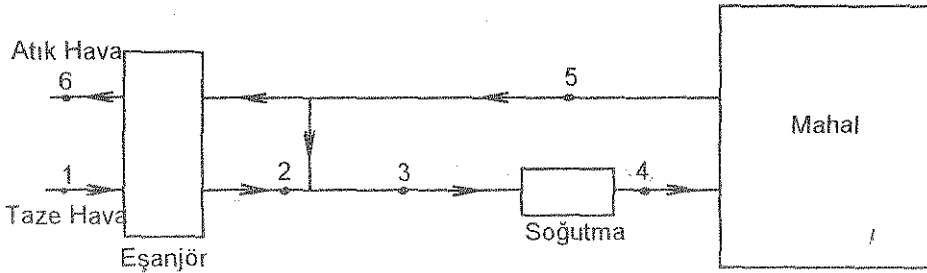
Şekil 15. Isı geri kazanımlı nemlendiricisiz yaz kliması
