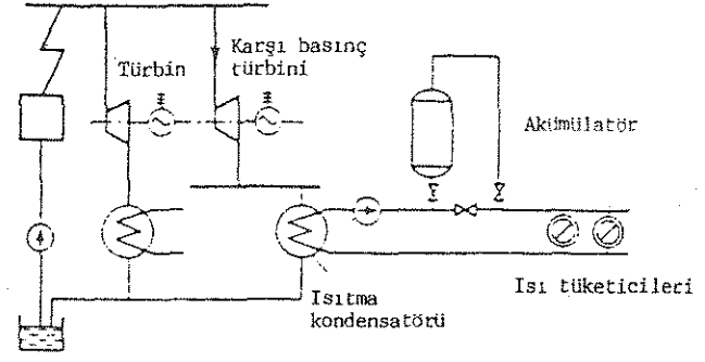
b) KARŞI BASINÇ TÜRBİNİ VE SICAK SULU BÖLGESEL ISITMA ŞEBEKESİ
