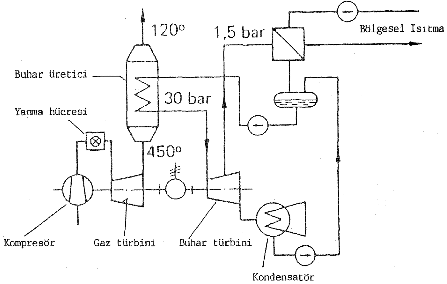
OMBİNE GAZ TÜRBİNLİ VE BUHAR TÜRBİNLİ DÜVET SANTRALİ ve BÖLGESEL İSITMA
