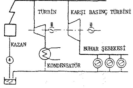
a) KARŞI BASINÇ TÜRBİNİ VE BUHAR ŞEBEKESİ
