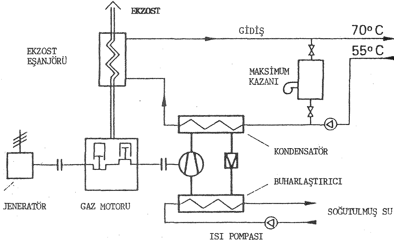
BLOK ISITMA VE KUVVET SANTRALİ'NİN ISI POMPASI İLE KOMBİNASYON
