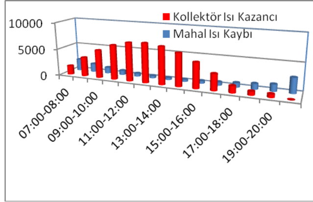
Şekil 5. Ekim Ayı Mahal Isı Kaybı-Kollektör Isı Kazancı Grafiği
