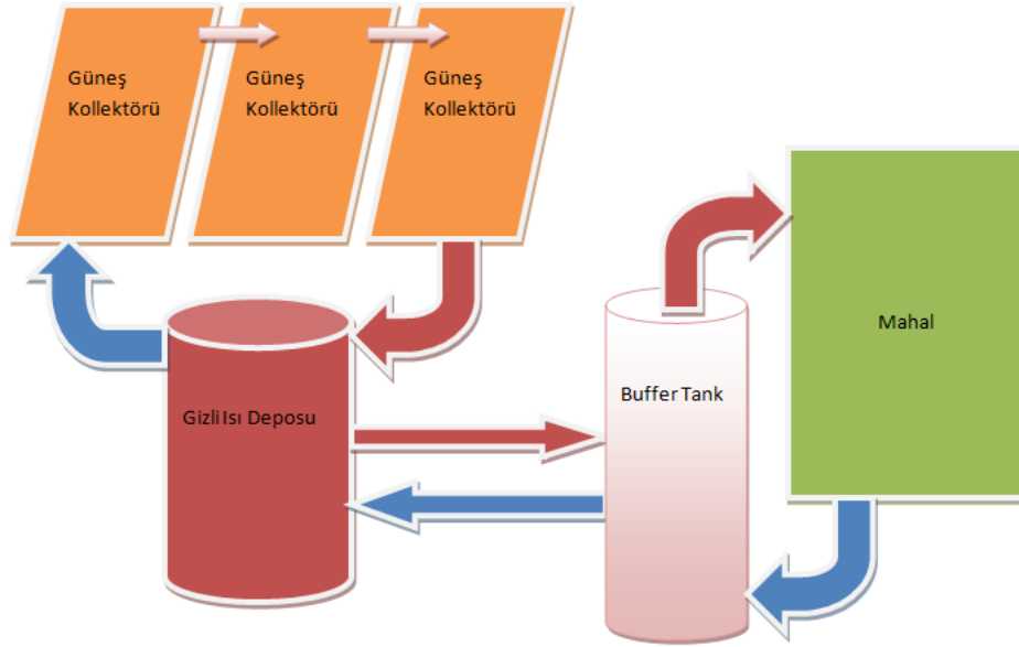
Şekil 4. Yıldız Yenilenebilir Enerji Evi Isıtma Sistemi Şeması
