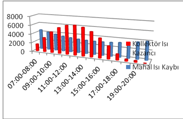
Şekil 10. Mart Ayı Mahal Isı Kaybı-Kollektör Isı Kazancı Grafiği
