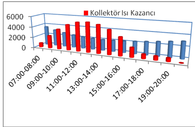
Şekil 6. Kasım Ayı Mahal Isı Kaybı-Kollektör Isı Kazancı Grafiği
