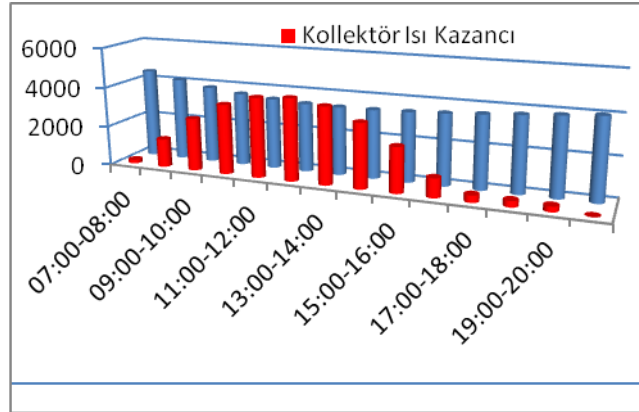
Şekil 7. Aralık Ayı Mahal Isı Kaybı-Kollektör Isı Kazancı Grafiği
