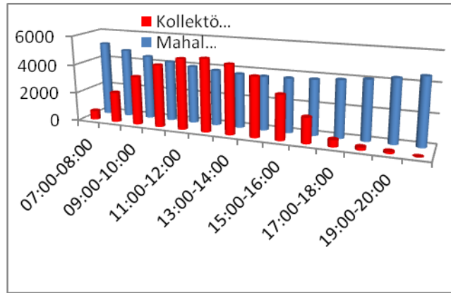
Şekil 9. Şubat Ayı Mahal Isı Kaybı-Kollektör Isı Kazancı Grafiği
