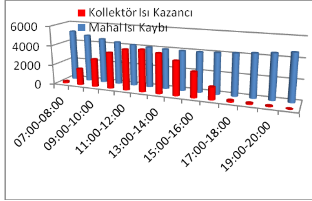
Şekil 8. Ocak Ayı Mahal Isı Kaybı-Kollektör Isı Kazancı Grafiği
